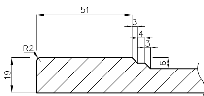
przekrój
