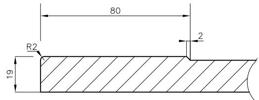
przekrój
