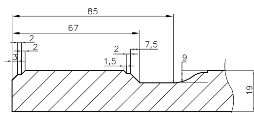
przekrój
