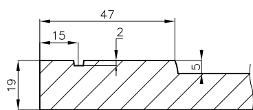
przekrój
